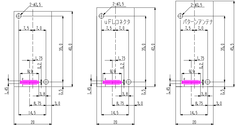
TWE-001-IP/PA ヘッダ (AXT440124)
