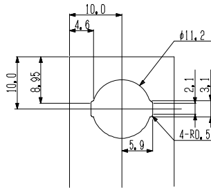
GY111B099-006アンテナホルダー取付穴(φ11.2)参考図
