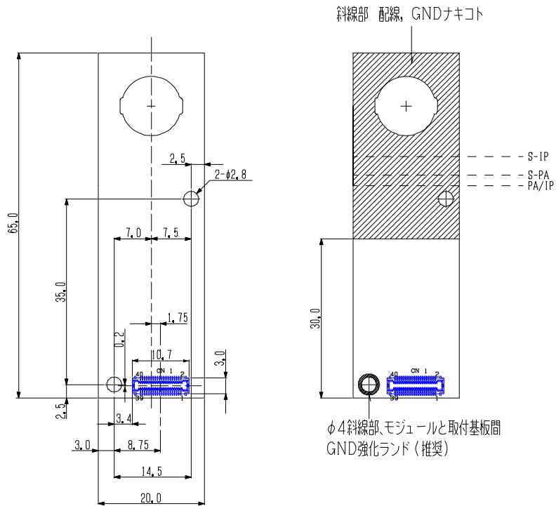
取付基板(参考図) 20×65×1.0t 受け側ソケット (AXT340224)
