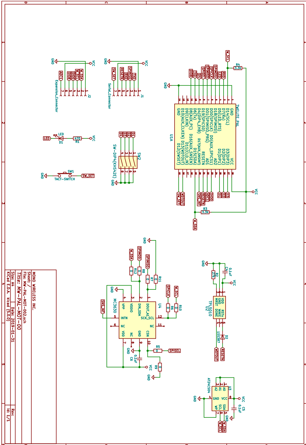
図 3 回路図
