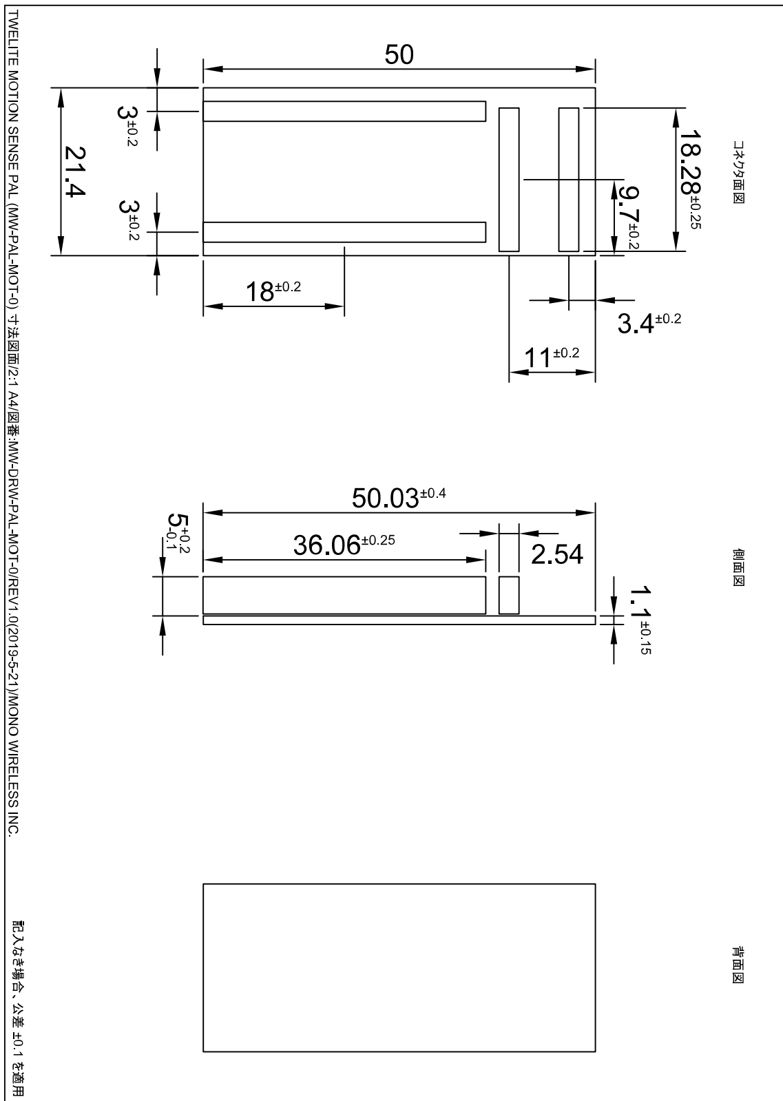
図 2 外形寸法図
