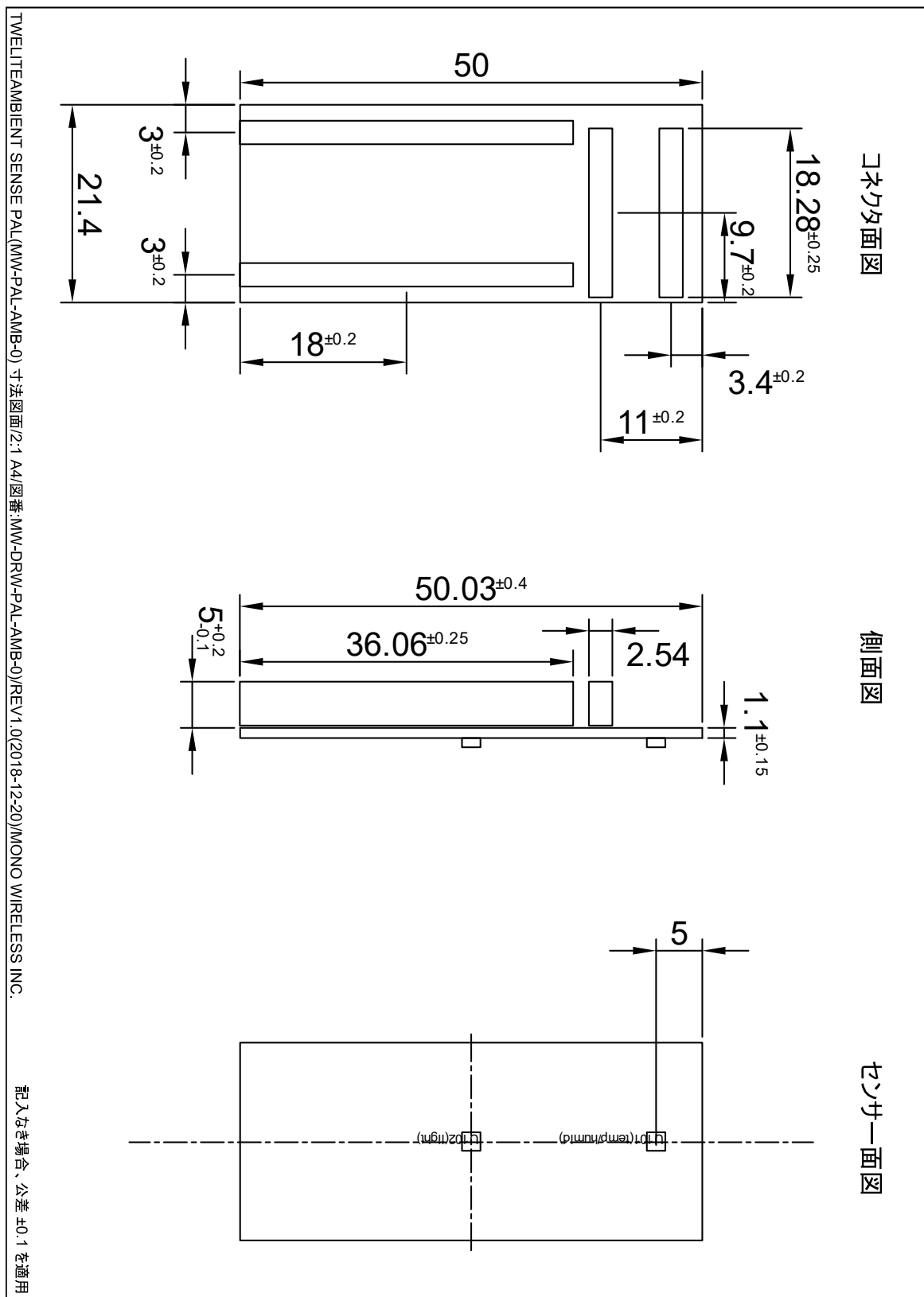
図 2 外形寸法図
