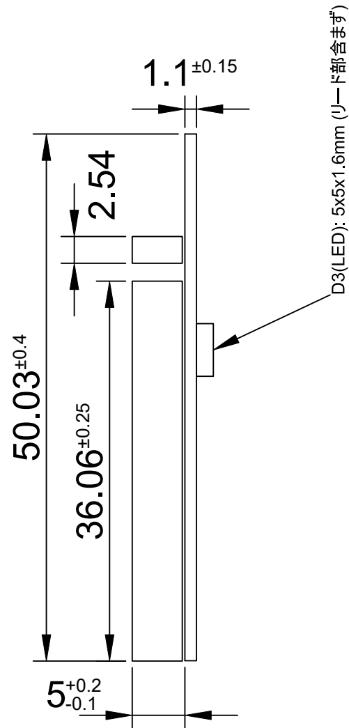
側面図
