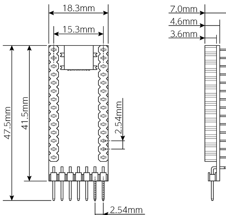
図 1 外形図
