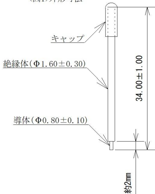
〈図1〉外形寸法
