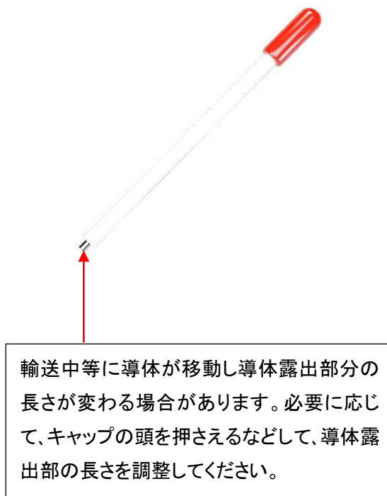
〈図2〉3D図
