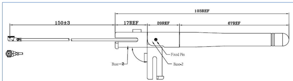
アンテナ寸法
